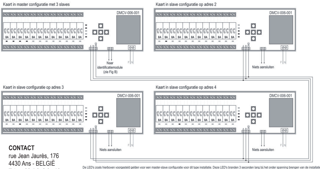
FIGUUR C - Verbinding van de DMCV-006-001 - Voorbeeld van een verbinding met 4 kaarten
