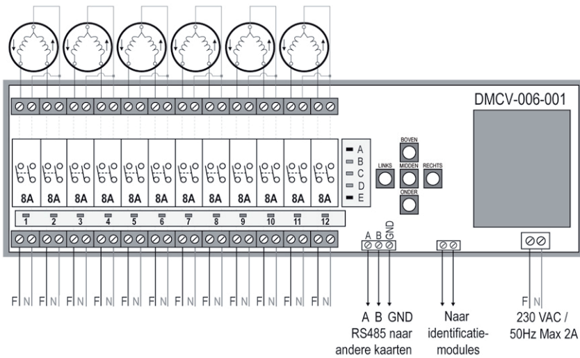
FIGUUR A - DMCV-006-001 kaart
